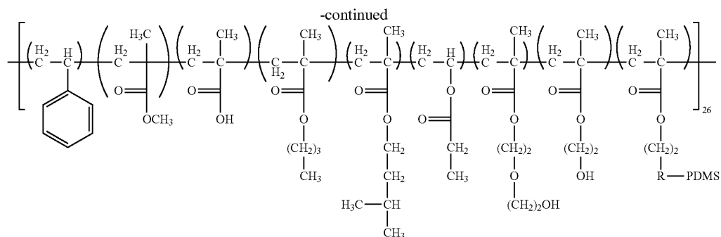
P[(S-MMA-MAA-BMA-iPMA-VP-HEGEMA-HEMA)-g-PDMS] 26
